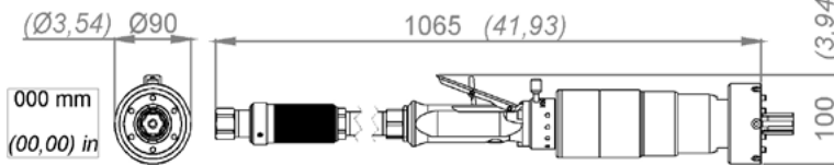
HL83S
